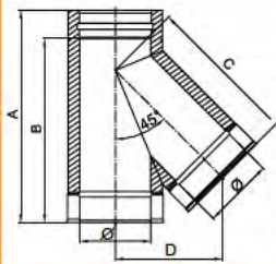
Tee 135° / 45° / DWECO - 12
