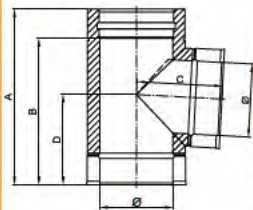
Tee 87° / DWECO - 1055
