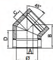
Elbow 45° / DWECO - 18
